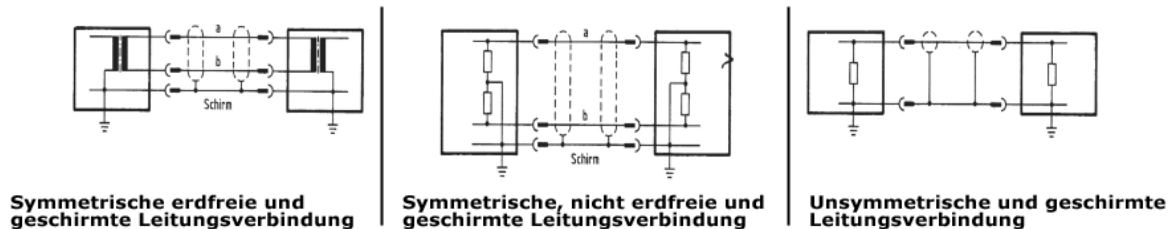
Abbildung 1.12: Symmetrische und unsymmetrische Signalführung. [Handbuch der Tonstudiotechnik II, S.91]
